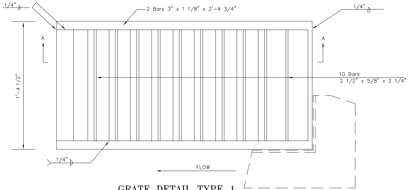
GRATE DETAIL TYPE 1 PLAN N.T.S.
